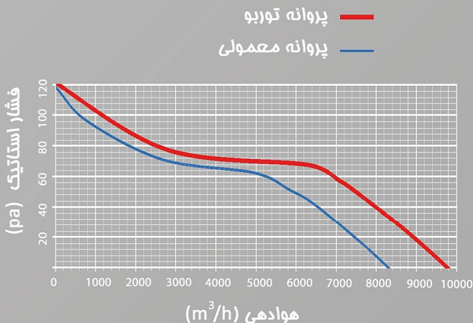
نمودار فن (هوادهی / فشار استاتیک) (مقایسه بلور معمولی و توربو)
